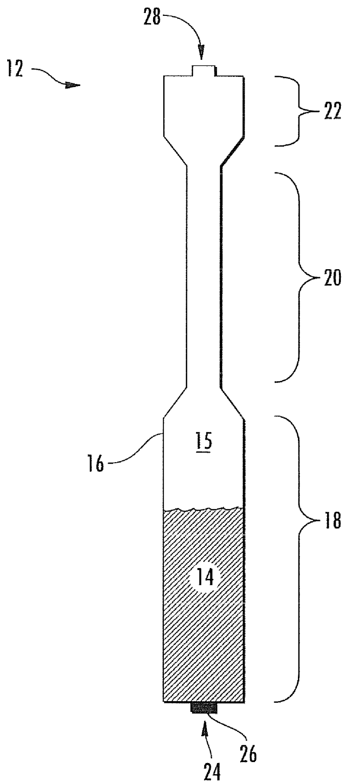
FIG. 1B
